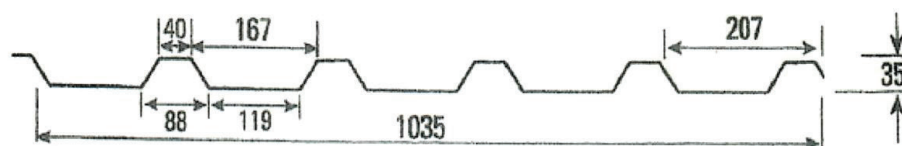
Abbildung 2: Querschnitt des Trapezprofils W35/1035
